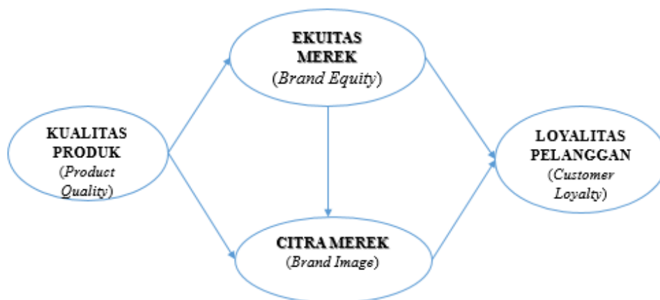
Gambar 2 Kerangka Pemikiran
